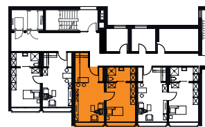
Grundriss des Hauses – 7. Obergeschoss
